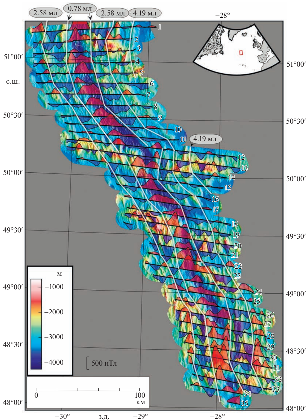
Рис. 4. Карта графиков аномального магнитного поля, наложенная на карту рельефа дна на полигоне Фардей. Цифрами обозначены номера профилей съемки, белые линии – изохроны, цифры в овалах – возраст литосферы, согласно выделенным линейным магнитным аномалиям.
