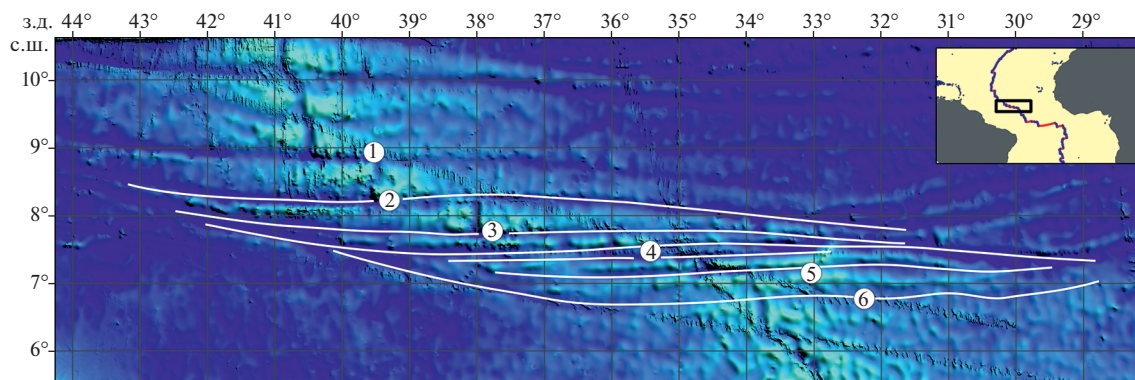
Рис. 1. Строение океанического дна в районе мегатрансформа Долдрамс (по данным [26]).
