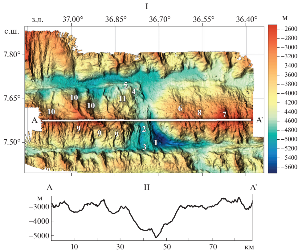
Рис. 5. Рельеф дна в районе спредингового сегмента СС-3 между разломами Вернадского и Пушаровского. I — батиметрическая карта (справа — шкала глубин), положение батиметрического профиля А—А' (линии белым), морфоструктуры (арабские цифры); II — батиметрический профиль А—А'.
