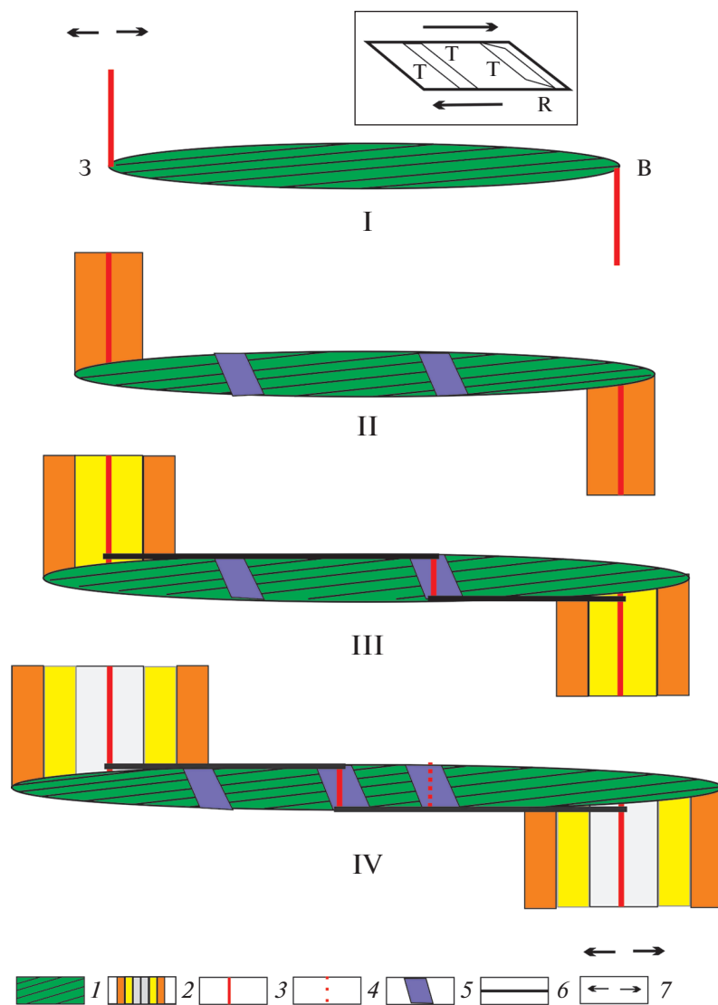
Рис. 11. Схема тектонического развития межразломного пространства двойного разлома Пушаровского.
